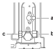
a Flüssigkeits-Absperrventil b Gas-Absperrventil c Service-Stutzen
