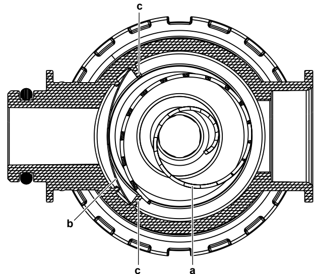
a Aufgerollter Filter b Sieb c Vorsprung
